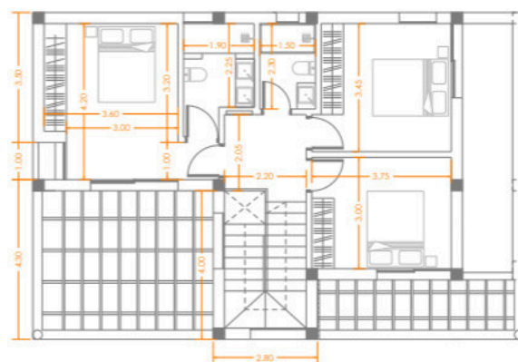
ΚΑΤΟΨΗ ΟΡΟΦΟΥ
