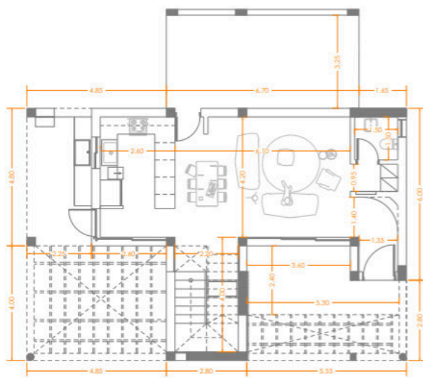
ΚΑΤΟΨΗ ΙΣΟΓΕΙΟ
